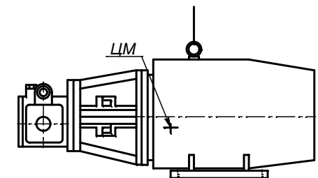
Схема строповки
